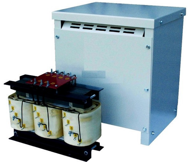
Encapsulado el gabinete metálico Plancha LAF y el horno texturizado (5kva - 2000kva)
